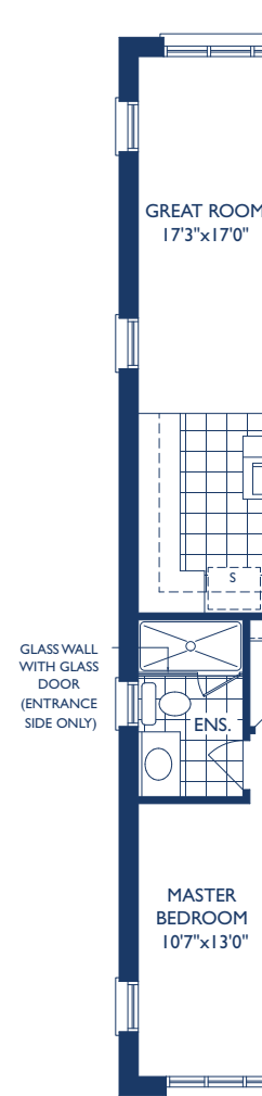
END ELEV. A
